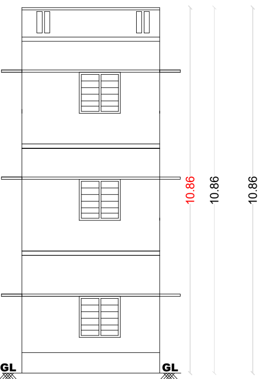
ELEVATION
