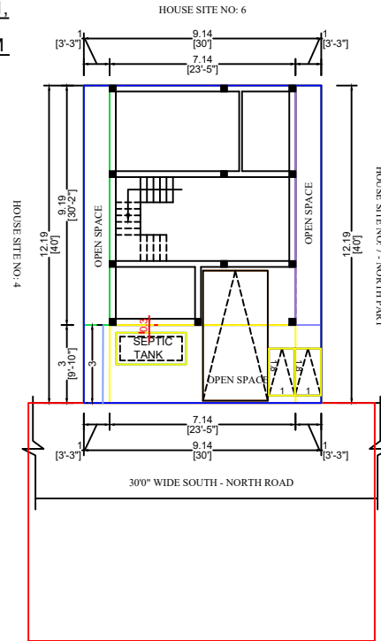
SITE PLAN SCALE 1:1
