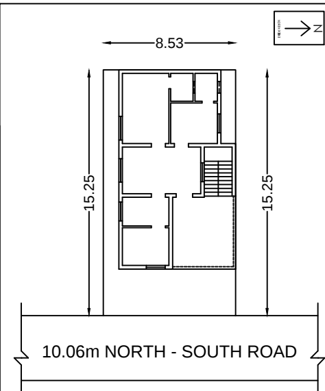
SITE PLAN : 1:150
