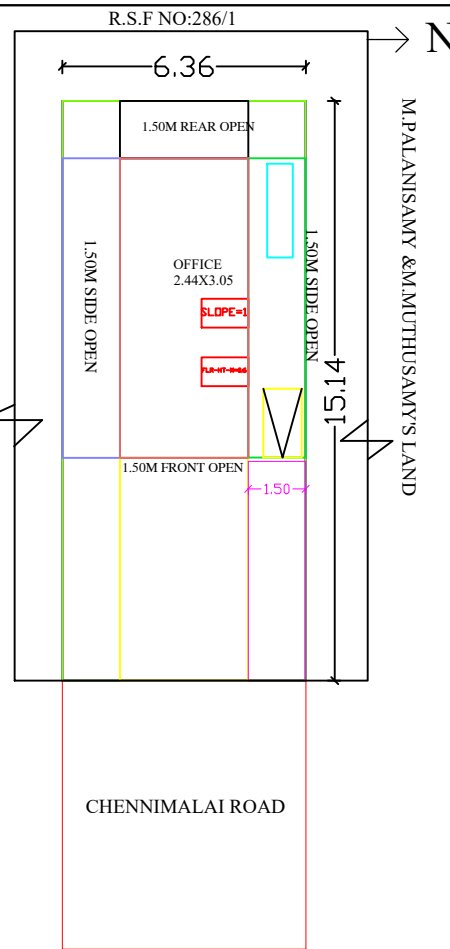
SITE PLAN SCALE 1:100
