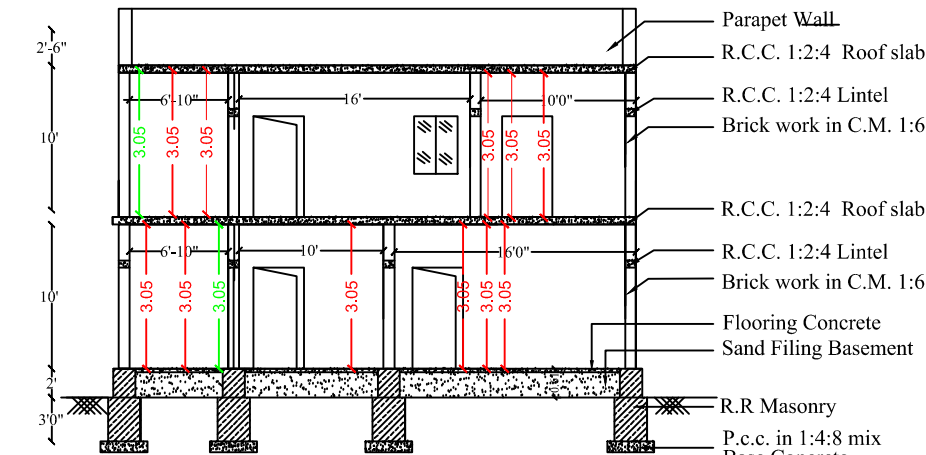
SECTION A-A
