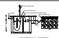
LONGITUDINAL SECTION
