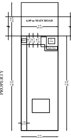
SITE PLAN ( Scale : 1:100)
