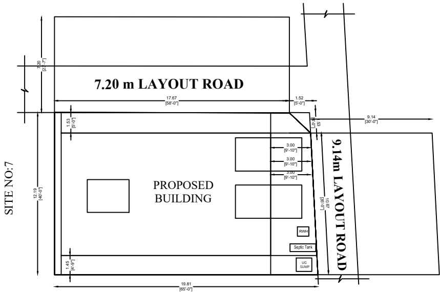
SITE NO:9 SITE PLAN ( Scale : 1:100)
