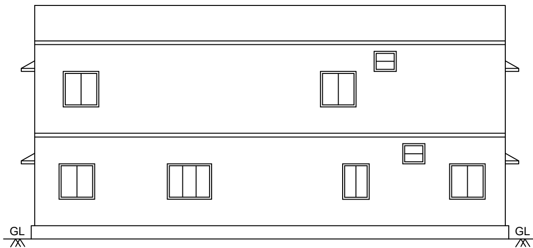
ELEVATION
