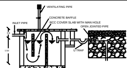
LONGITUDINAL SECTION
