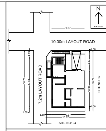
SITE PLAN : 1:200
