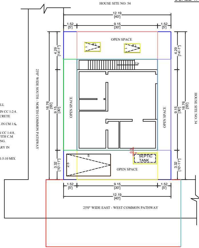
SITE PLAN SCALE 1:1
