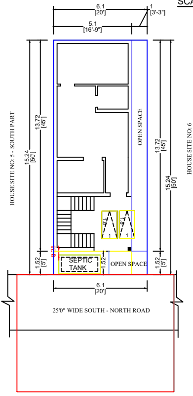
SITE PLAN SCALE 1:1
