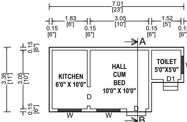
PLAN ( SCALE 1 : 100 )
