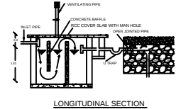
LONGITUDINAL SECTION
