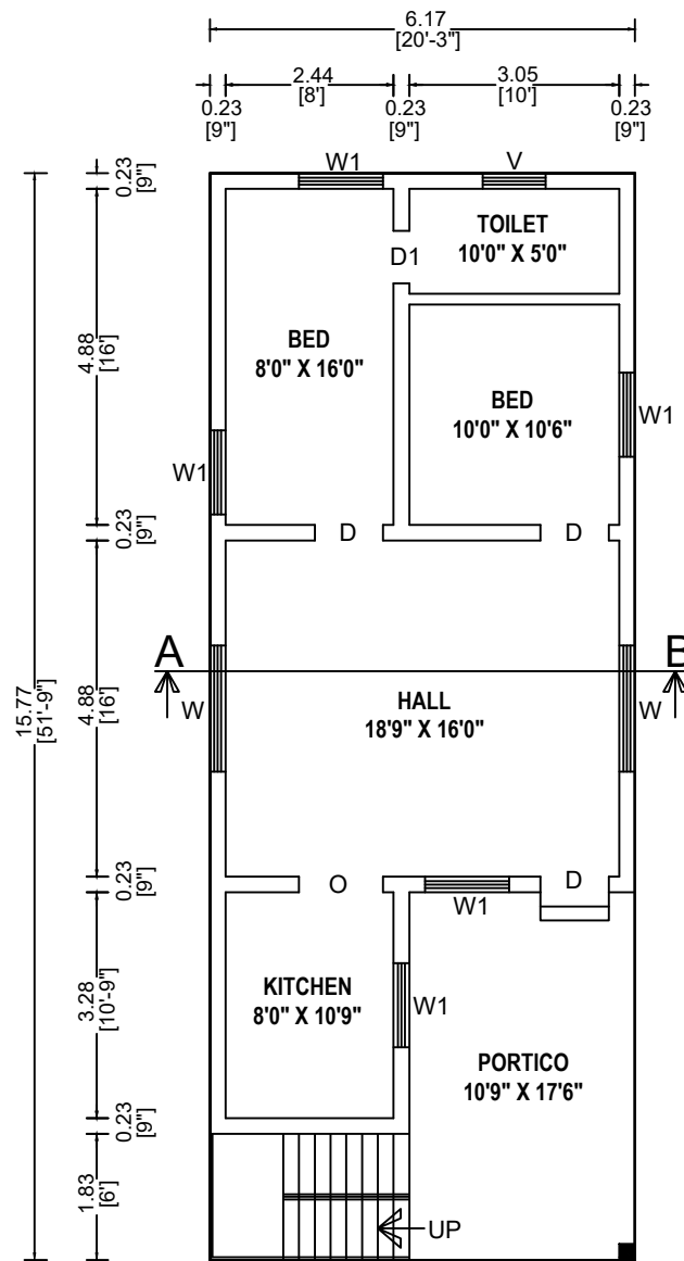
PLAN ( SCALE 1 : 100 )
