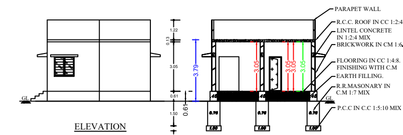
ELEVATION
