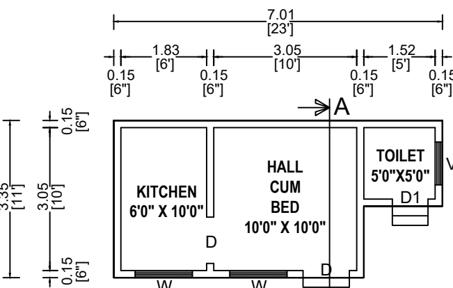
PLAN ( SCALE 1 : 100 )
