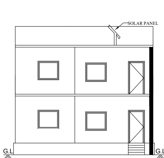
ELEVATION
