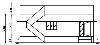
ELEVATION
