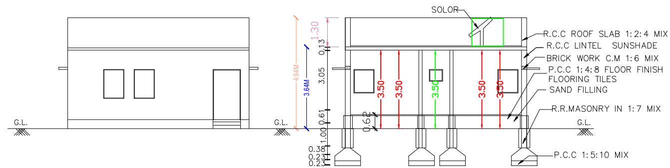
ELEVATION
