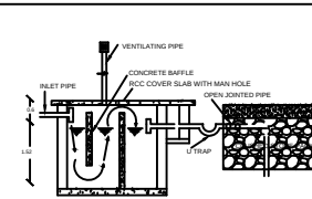
LONGITUDINAL SECTION
