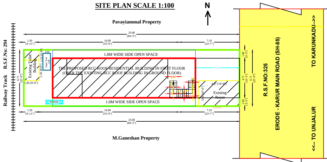
SITE PLAN SCALE 1:100
