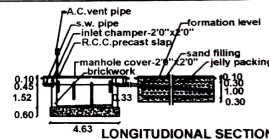
LONGITUDINAL SECTION
