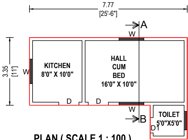
PLAN ( SCALE 1 : 100 )
