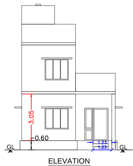
ELEVATION
