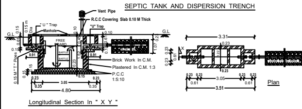
Longitudinal Section in " X Y "
