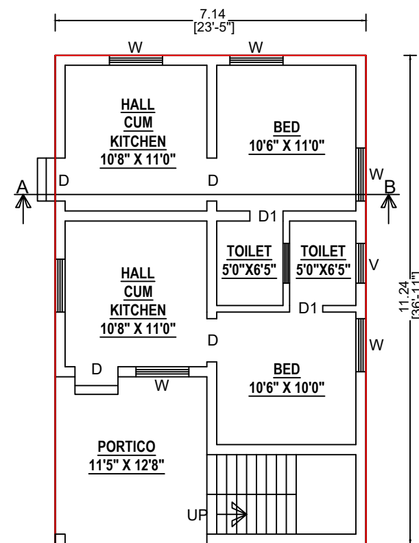
PLAN (SCALE 1 : 100)
