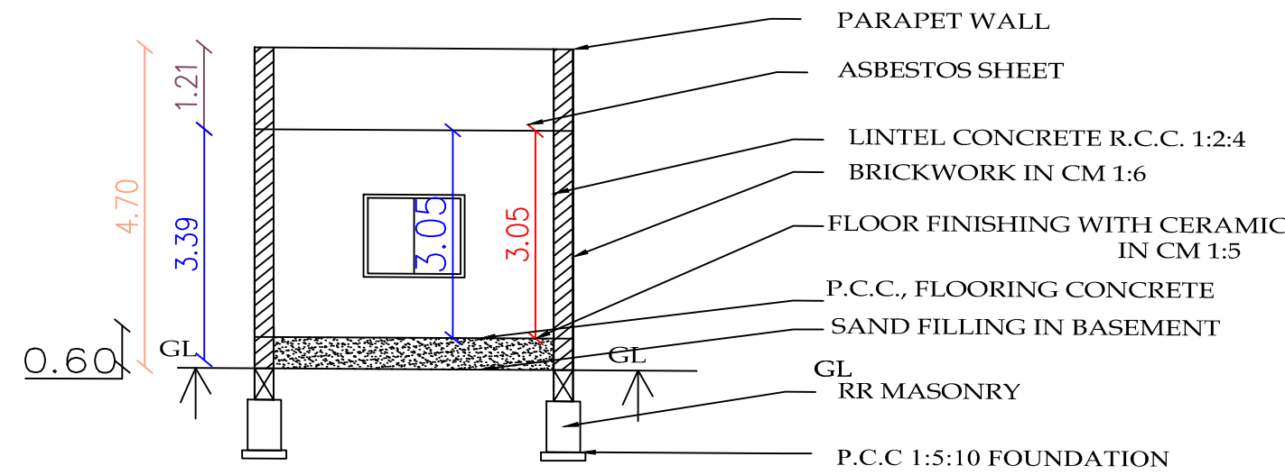
SECTION A-A
