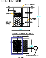
LONGITUDINAL SECTION
