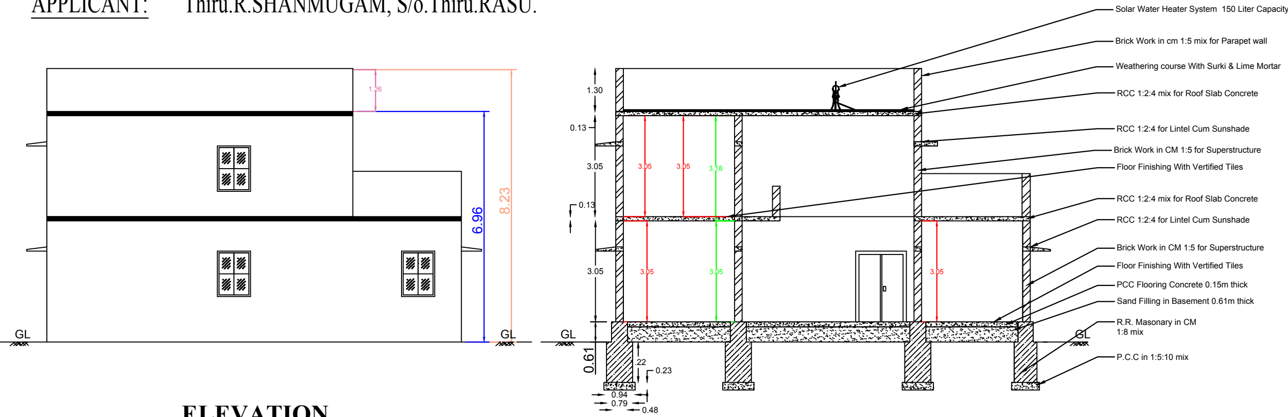
ELEVATION
