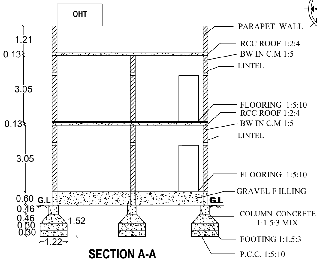
SECTION A-A
