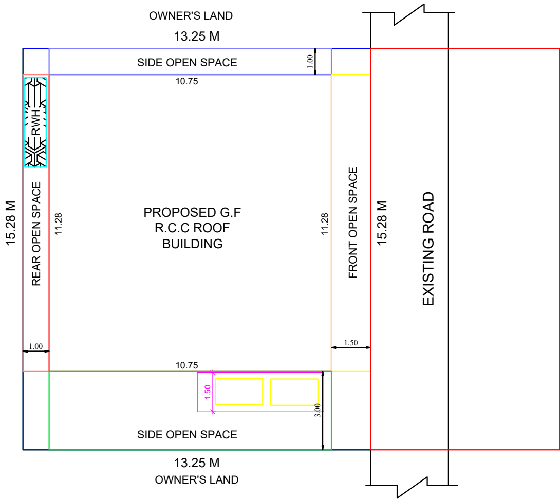
SITE PLAN SCALE 1CM : 1M
