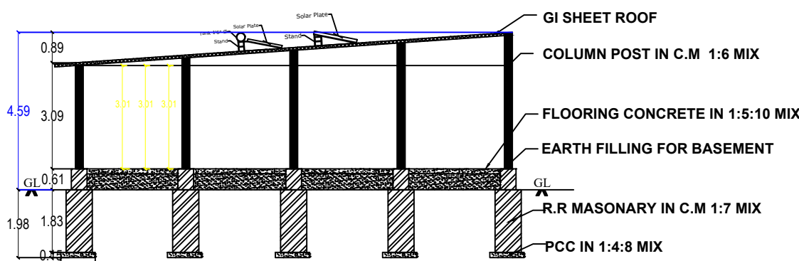
SECTION 'AB'
