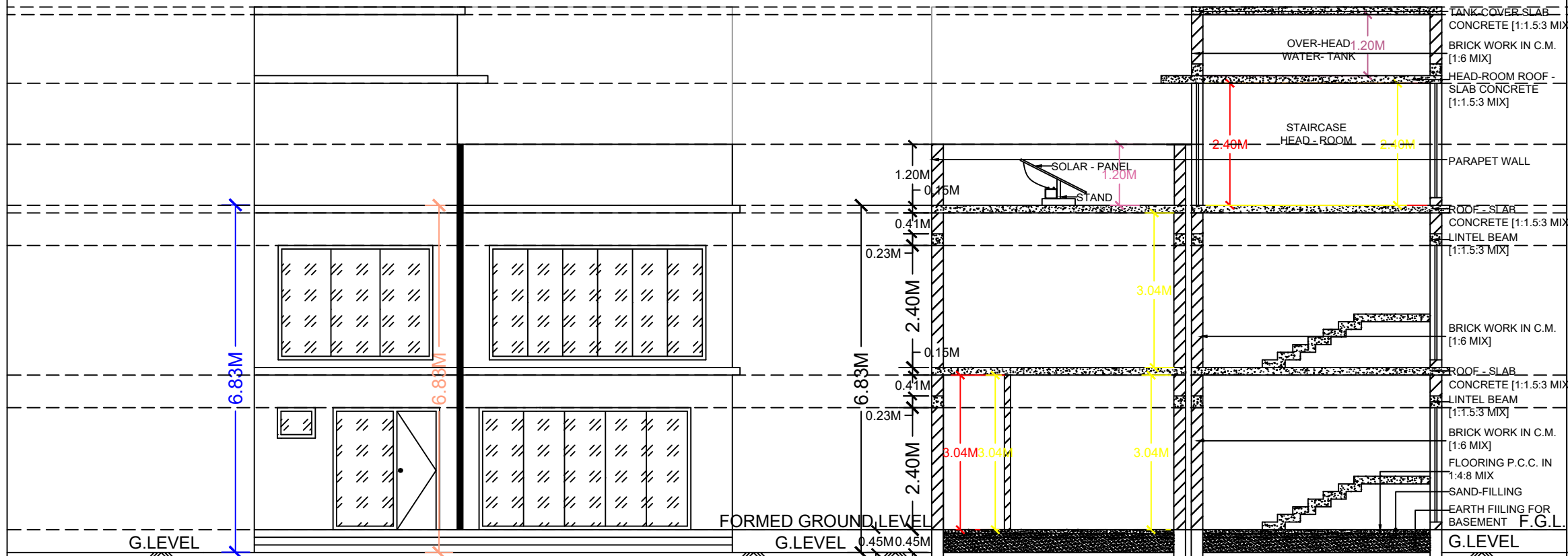
ELEVATION
