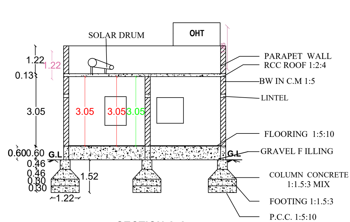
SECTION A-A
