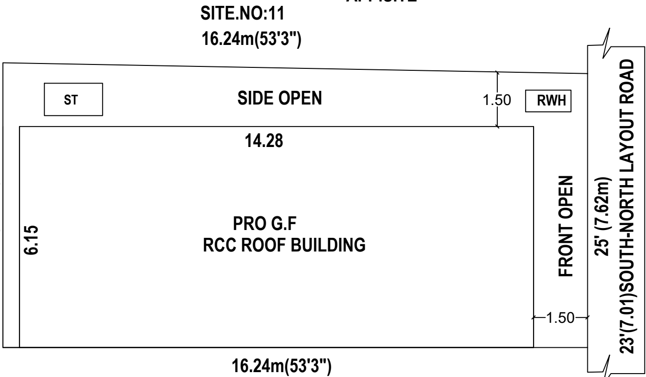
SITE NO:12 A SITE PLAN
