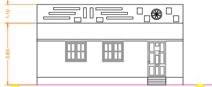
ELEVATION - A
