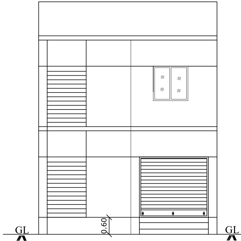
ELEVATION
