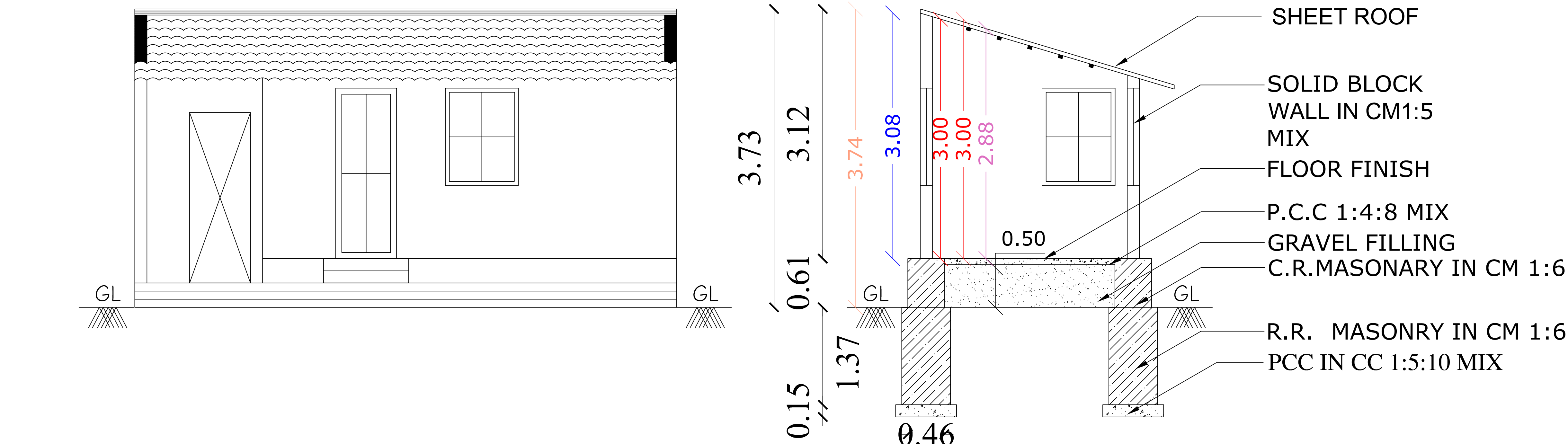
ELEVATION
