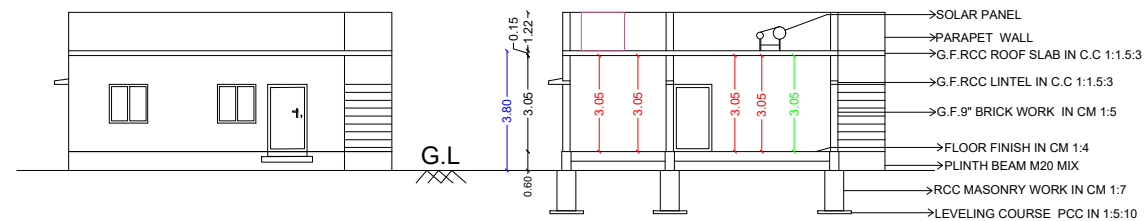
ELEVATION
