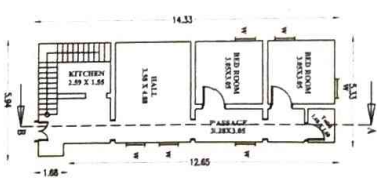
ACTUAL GROUND FLOOR PLAN
