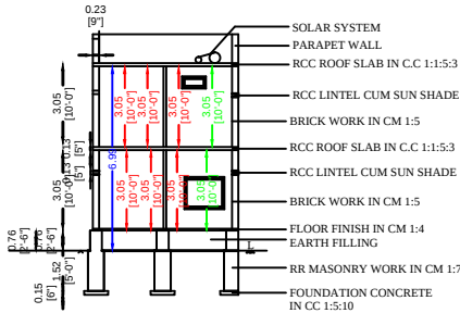
SECTION "AA", "BB"
