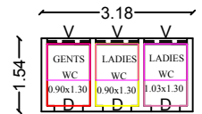
TOILET PLAN
