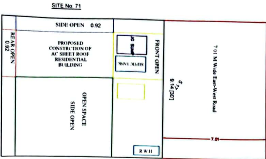
SITE PLAN 1:100
