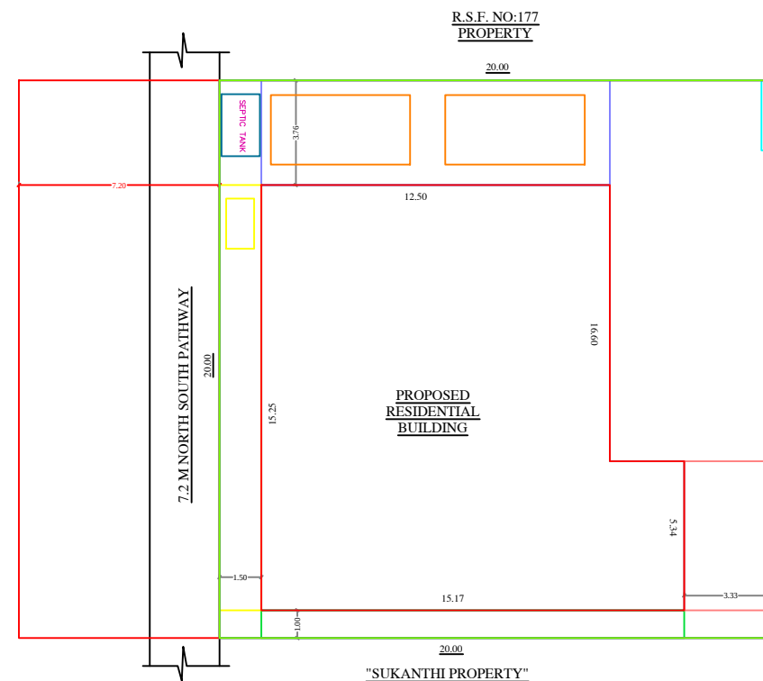
SITE PLAN 1:100
