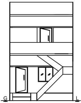
ELEVATION
