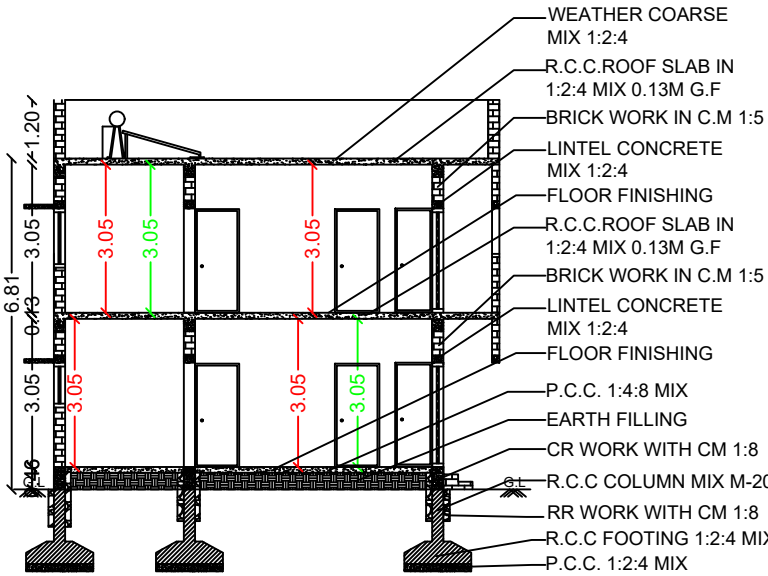
SECTION - AB
