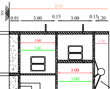
SECTION A-B
