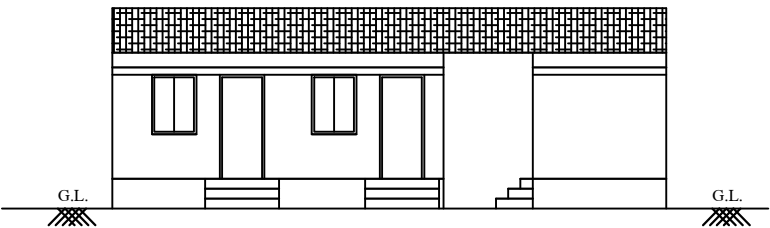
ELEVATION
